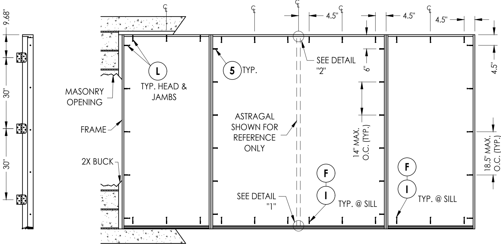
HINGE JAMB
